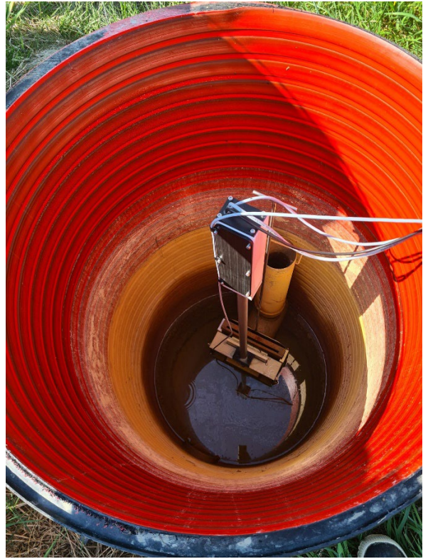
Kuva 11. Peltosäätö -hankkeessa testattua automaattikkaa salaojakaivossa Kannuksen pilottilohkolla.
